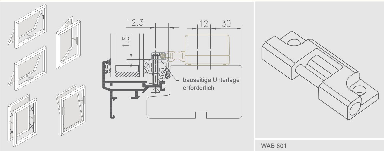
Montagevorschlag 4 - Auswärts öffnend
