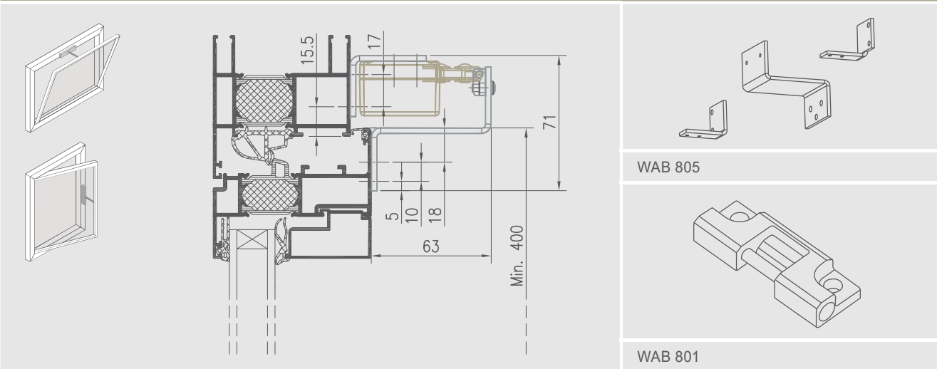
Montagevorschlag 3 - Einwärts öffnend
